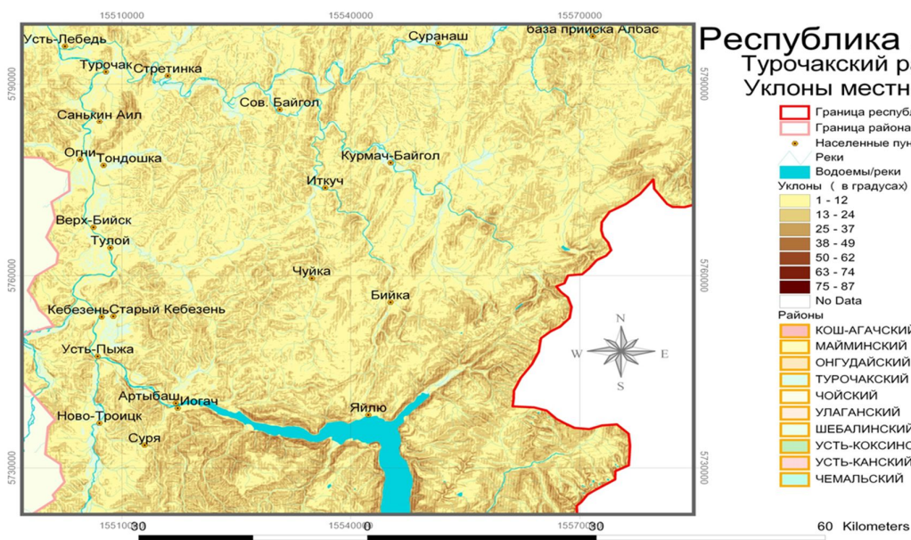
Рисунок 4 – Прототип твердой копии карты с уклонами местности
