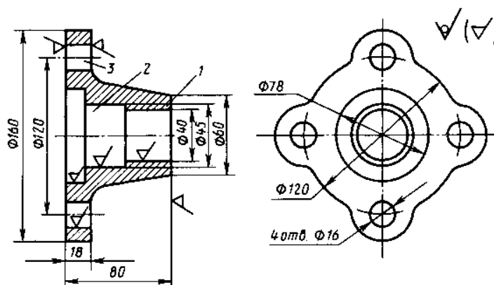
Вариант 6. Крышка Сталь 45. Производство массовое
