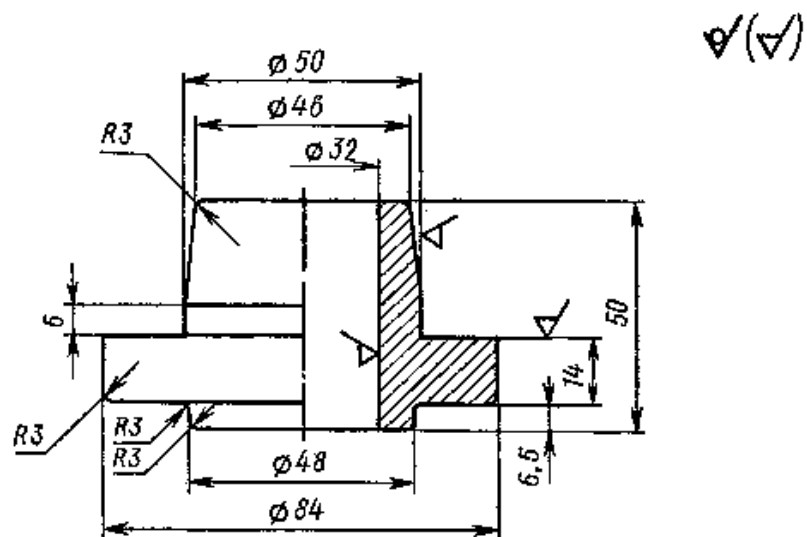
Вариант 3. Ступица Сталь 15. Производство массовое
