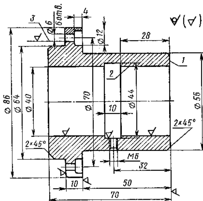
Вариант 5. Втулка Сталь 35. Производство единичное
