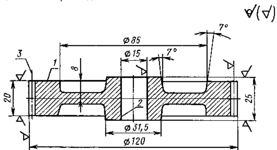
Вариант 3. Ступица Сталь 15. Производство массовое
