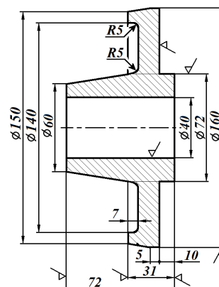
Вариант 2. Фланец
