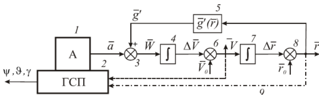
Рисунок 1 – Обобщённая схема платформенной инерциальной навигационной системы
