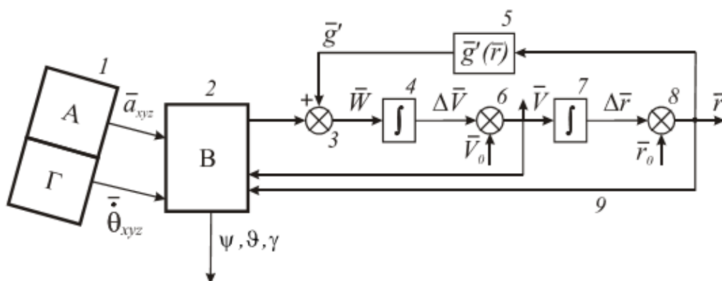
Рисунок 2 – Обобщённая схема безплатформенной инерциальной навигационной системы
