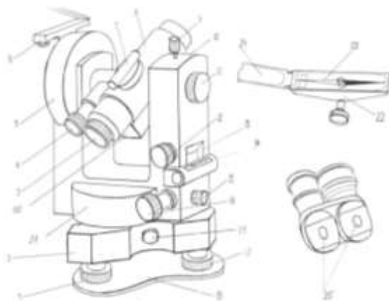
Рисунок 1 – Теодолит 4Т30
