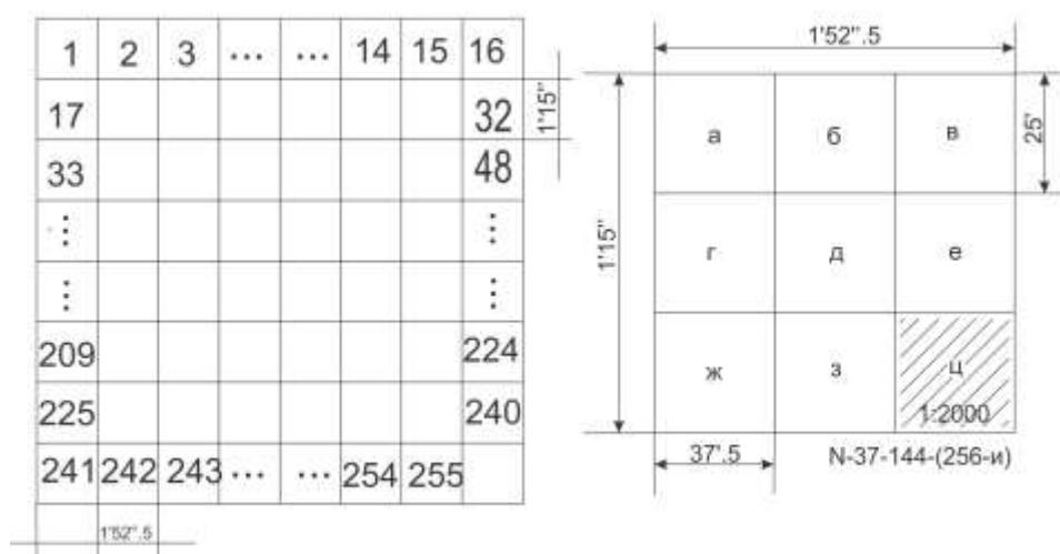
Рис. 3. Номенклатура листов планов масштабов 1: 5000 и 1: 2000
