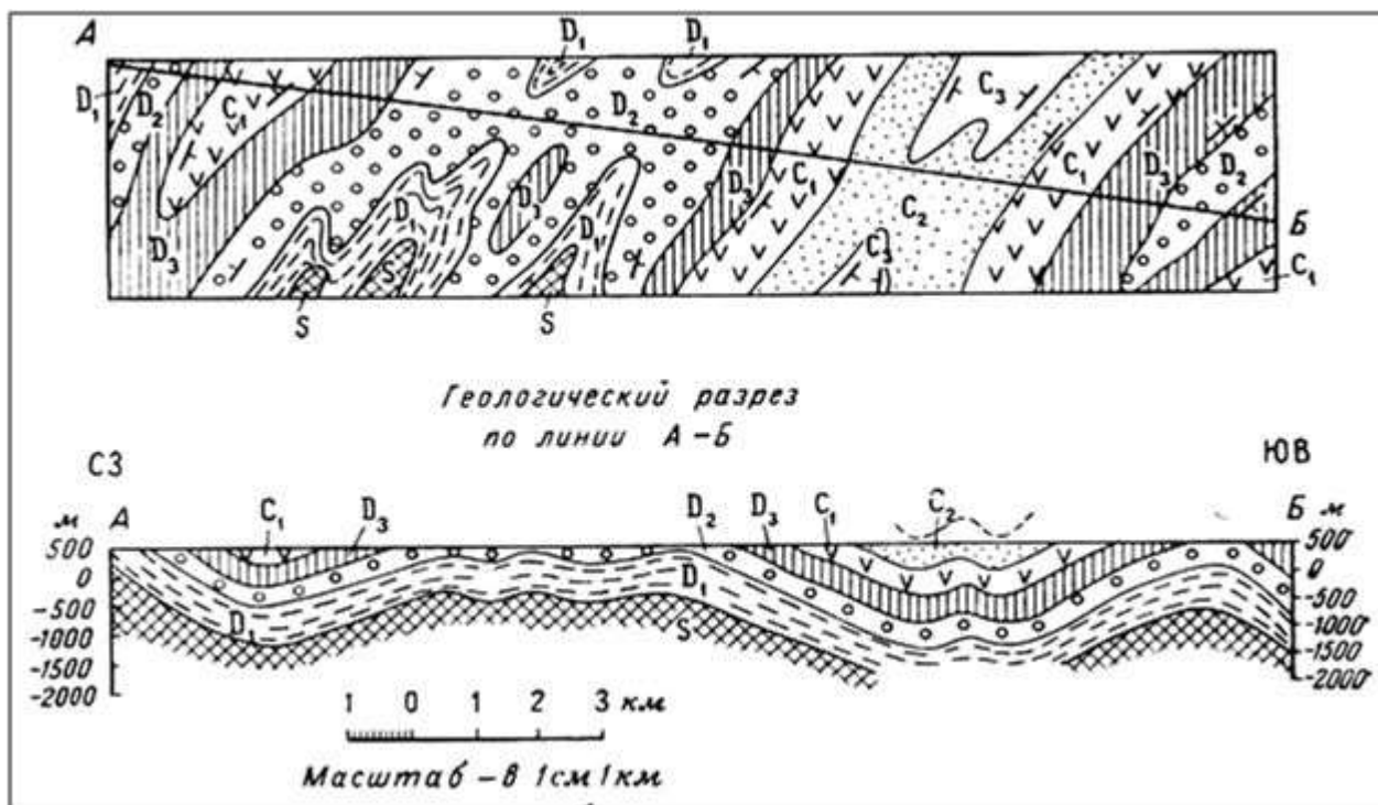
Рис. 1 – Геологический разрез по линии А-Б
