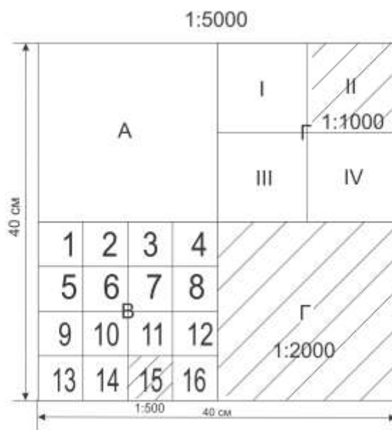
Рис. 4. Прямоугольная разграфка листа плана масштаба 1:5000
