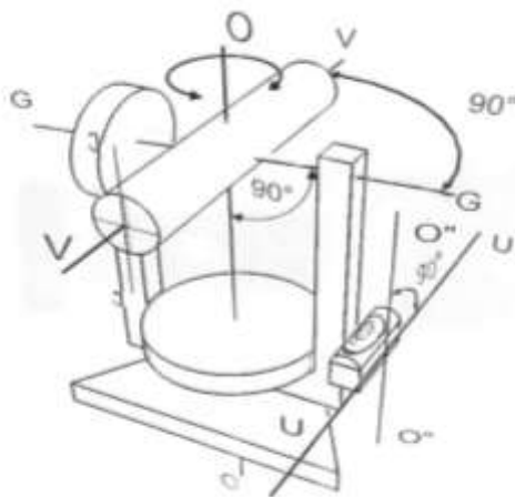
Рисунок 2 – Поверки теодолита 4Т30
