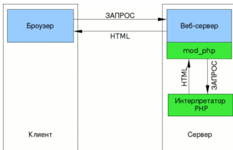
Рис. 1. Препроцессинг HTML на сервере
