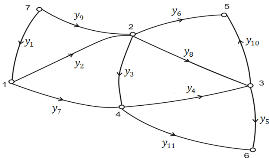
Рис 1. Нивелирная сеть
