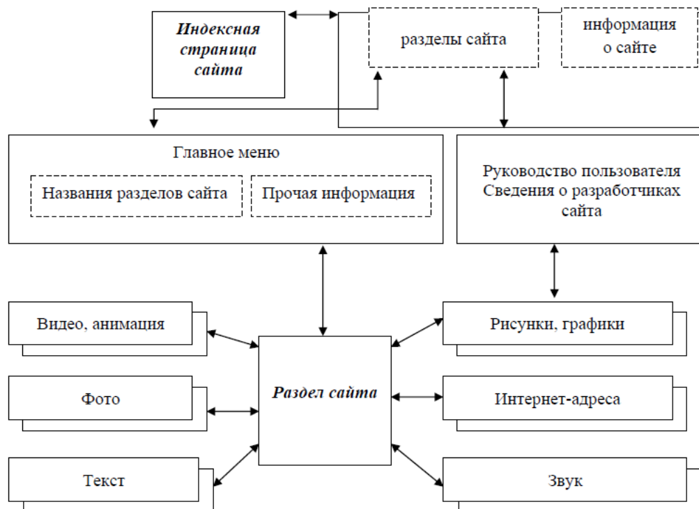
Рисунок 1 – Пример общей структуры сайта
