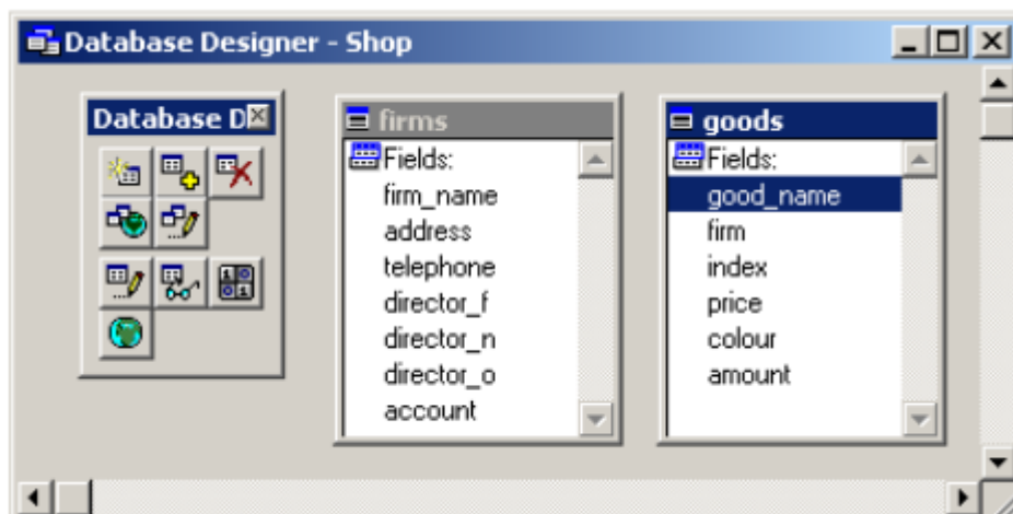
Рис.1. Окно конструктора базы данных с добавленными таблицами firms и goods
