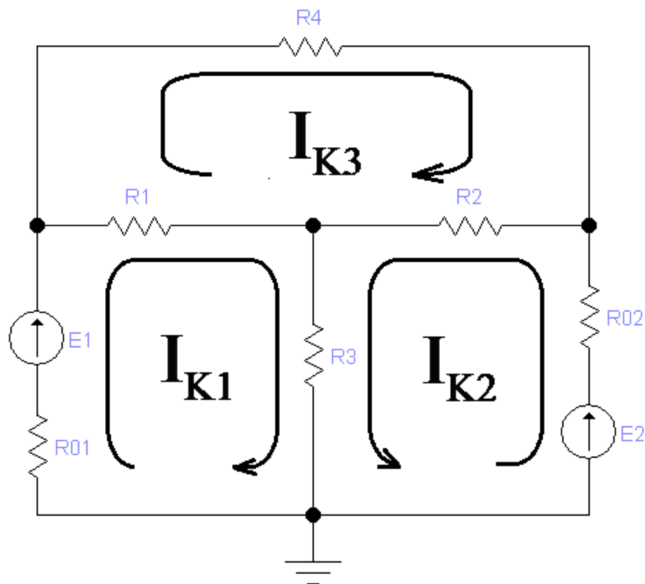
Рис.1 Исследуемая схема.
