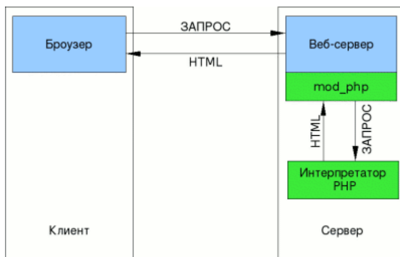
Рис. 1. Препроцессинг HTML на сервере
