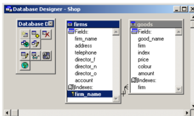
Рис. 2. Установка связи между таблицами
