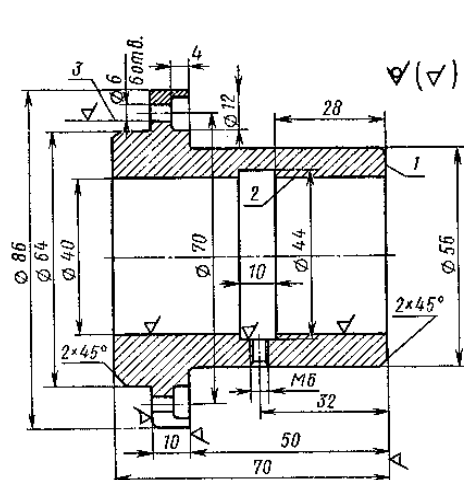
Вариант 1. Втулка
