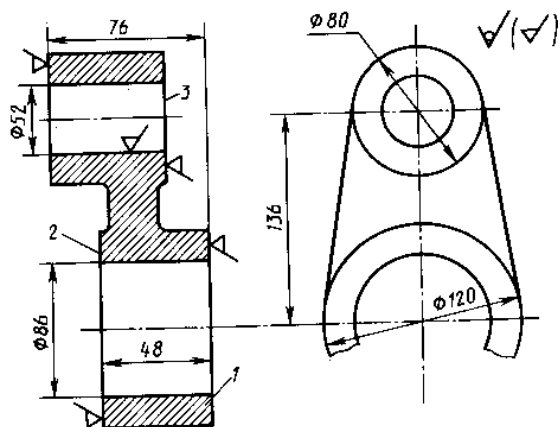
Вариант 1. Серьга
