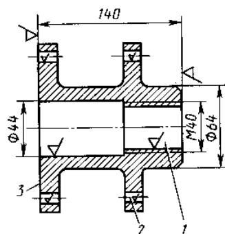
Вариант 1. Фланец
