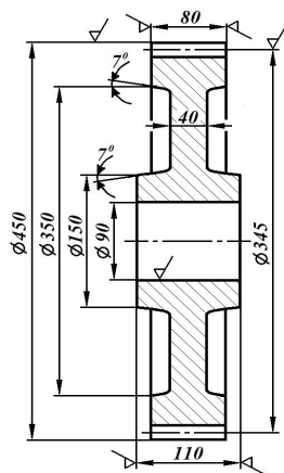
Вариант 1. Ступица
