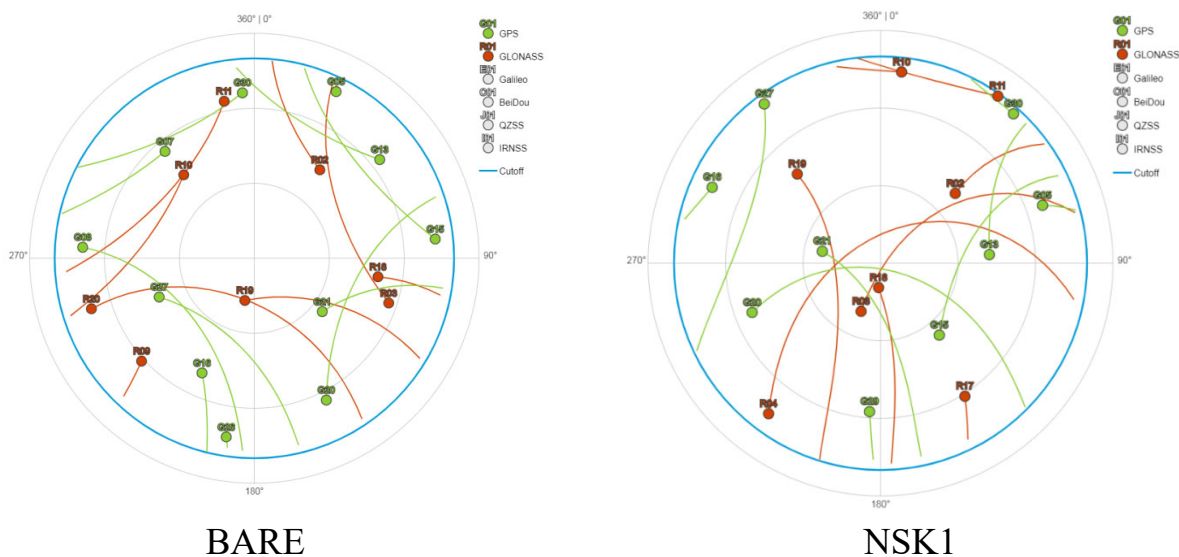
Рис. 2. Карта неба на пунктах BARE и NSK1 (02.01.2020), Trimble GNSS Planning
