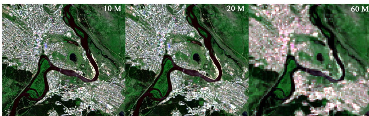
Рис. 3. Снимок на 19 июня с пространственными разрешениями 10 м, 20 м, 60 м
