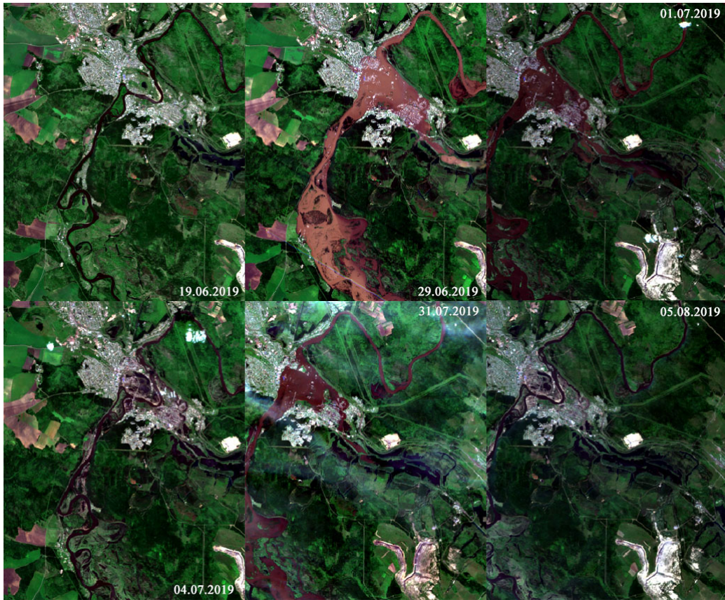
Рис. 4. Результат сшивки, обрезки области интереса и выбор каналов для дальнейшего анализа на каждую из дат
