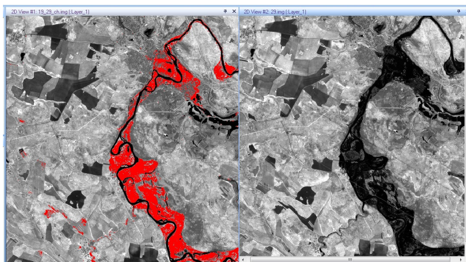
Рис. 7. Маска зон подтопления
