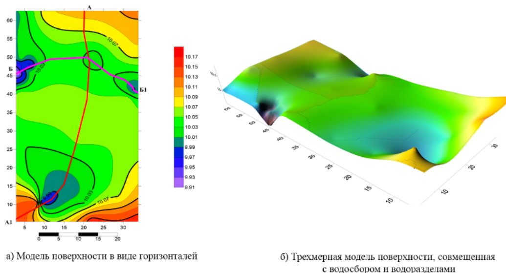
Рис. 3. Модели микрорельефа хоккейной коробки СГУГиТ
