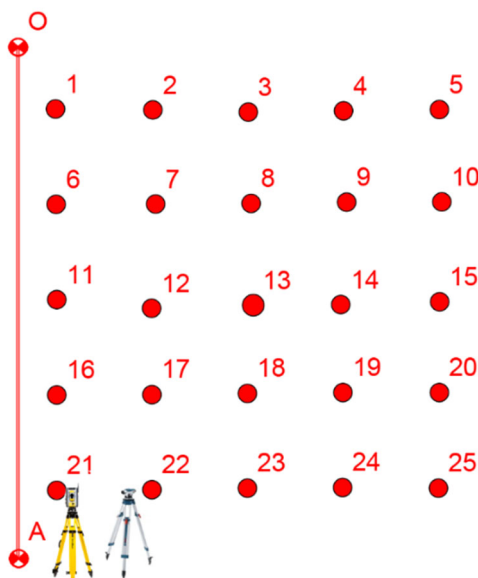
A – станция; 1–25 – съемочные точки
